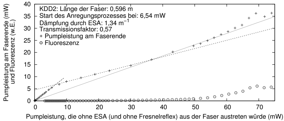
Abb. 4.8: Pumplichtabsorption und Fluoreszenz der Faser KDD2.
