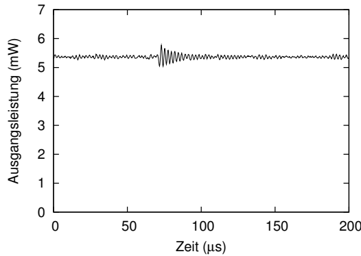
Abb. 3.15: LVF3c: Ausgangsleistung.
