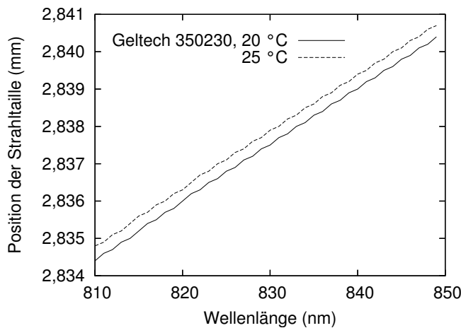
Abb. 3.12: Position der Strahltaille als Funktion der Wellenlänge für eine Linse vom Typ Geltech 350 230. (Die Daten wurden von Dr. Hünkemeier (unique-m.o.d.e AG) zur Verfügung gestellt.)
