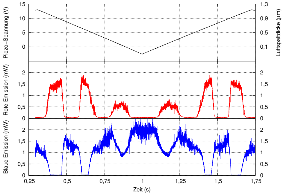
Abb. 5.7: Umschaltung der Emissionsfarbe durch Modulation des Abstandes des Auskoppelspiegels zur Faserendfläche, große Piezo-Amplitude.
