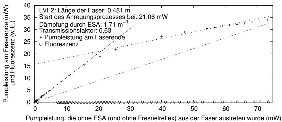
Abb. 4.9: Pumplichtabsorption und Fluoreszenz der Faser LVF2.
