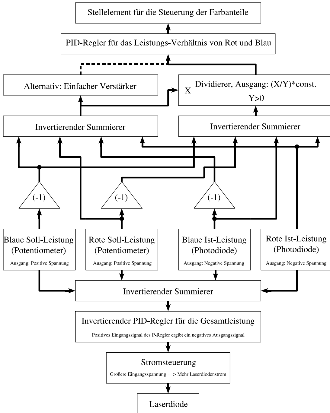
Abb. C.1: Blockschaltbild für die Leistungsstabilisierung.
