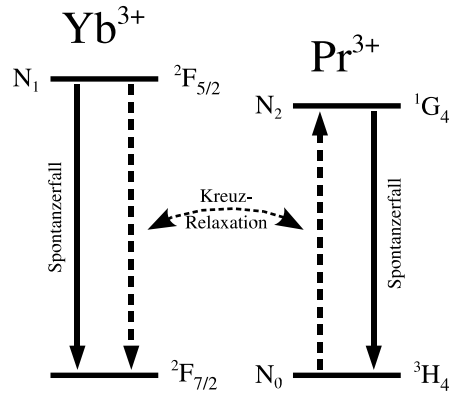
Abb. 4.21: Zerfall der Besetzung des ^1G_4 -Niveaus.
