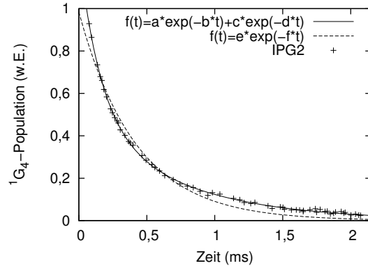
Abb. 4.20: Zerfall der Besetzung des ^1G_4 -Niveaus der Faser IPG2.
