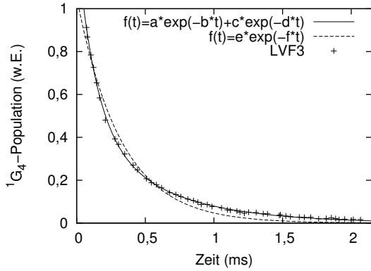
Abb. 4.19: Zerfall der Besetzung des ^1G_4 -Niveaus der Faser LVF3.
