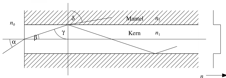
Abb. 2.1: Lichtführung in einer Stufenindexfaser.
