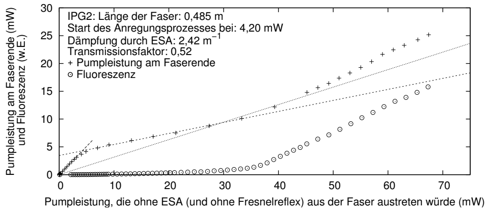
Abb. 4.7: Pumplichtabsorption und Fluoreszenz der Faser IPG2.
