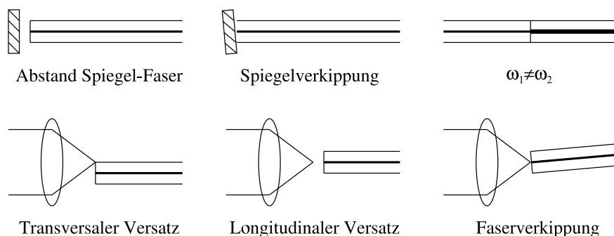
Abb. 3.5: Mögliche Justagefehler: Spalt zwischen Spiegel und Faser, Spiegel-Verkipfung und unterschiedlicher Modenfelddurchmesser zweier Fasern (oben). Transversaler bzw. longitudinaler Versatz des Pumplichtfokus und Verkipfung der Faser gegen die optische Achse des Pumplichtes (unten).
