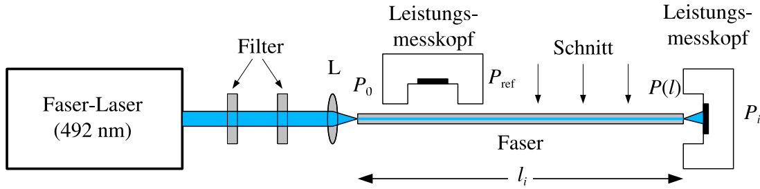
Abb. 4.2: Versuchsaufbau zur Bestimmung der Dämpfungsverluste bei 492 nm.
