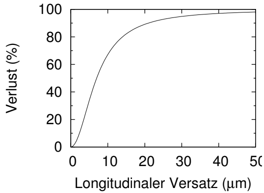
Abb. 3.8: Pumplichtverlust durch longitudinalen Versatz des Faserendes zum Pumplichtfokus.
