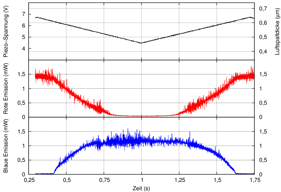
Abb. 5.8: Umschaltung der Emissionsfarbe durch Modulation des Abstandes des Auskoppelspiegels zur Faserendfläche, kleine Piezo-Amplitude.
