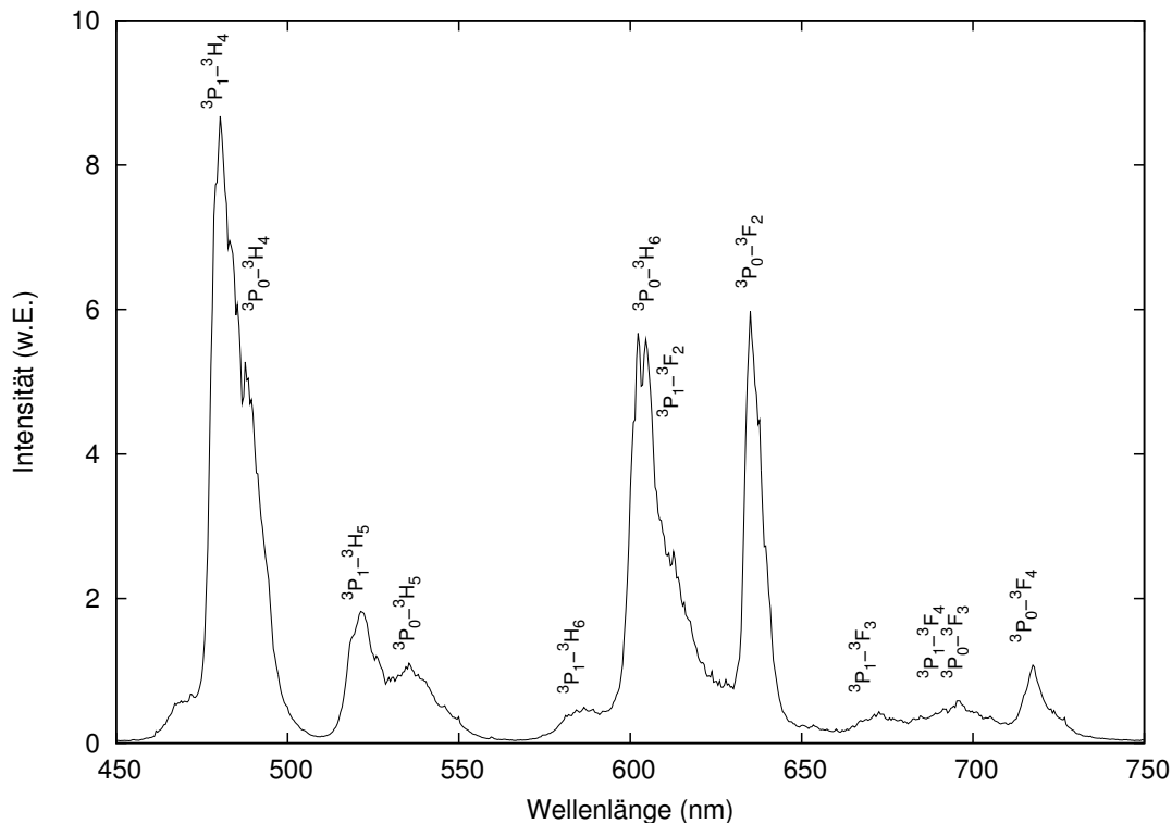
Abb. 2.9: Fluoreszenz-Spektrum der Faser LVF3b.
