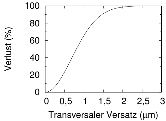
Abb. 3.9: Pumplichtverlust durch transversalen Versatz des Faserendes zum Pumplichtfokus.
